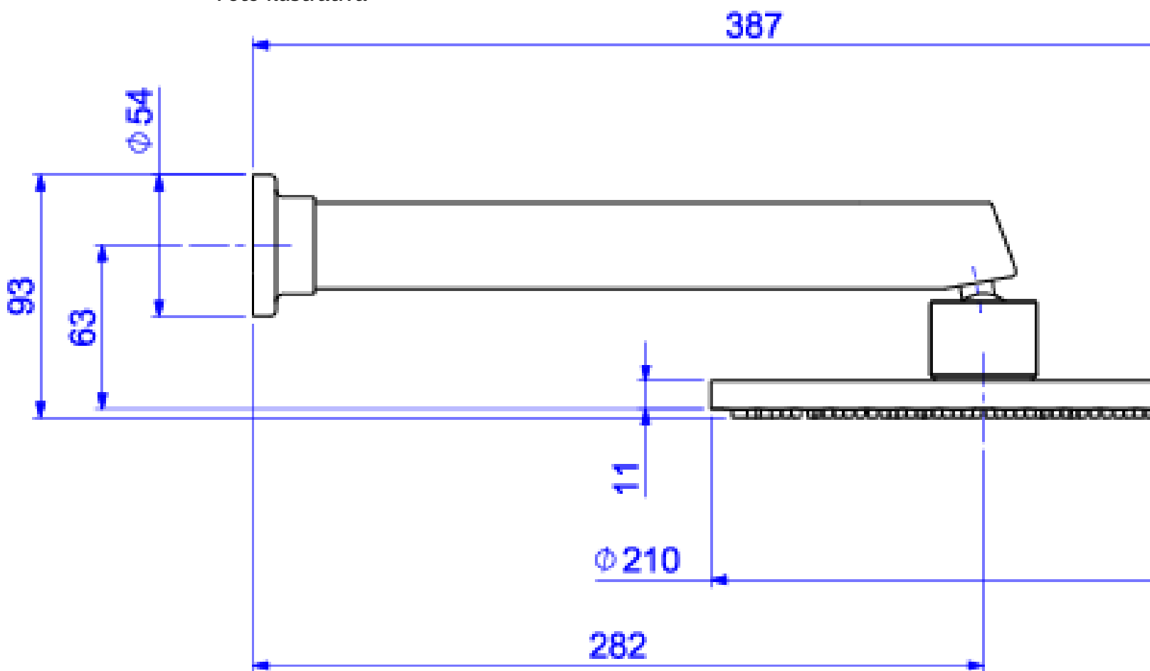
Desenho Técnico
