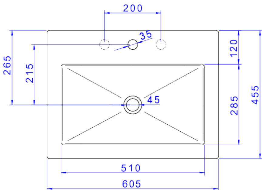
Desenho Técnico
