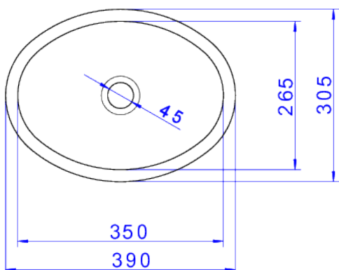
Desenho Técnico
