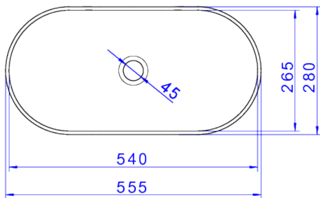
Desenho Técnico
